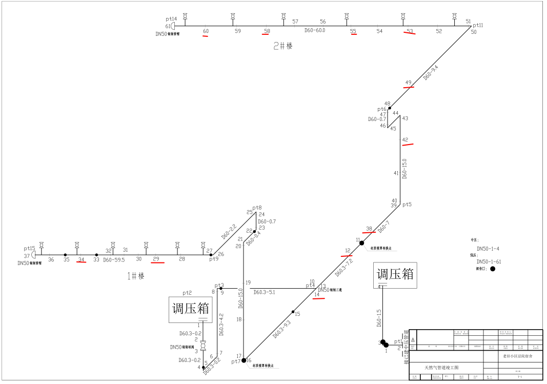
焊缝 焊缝-60
