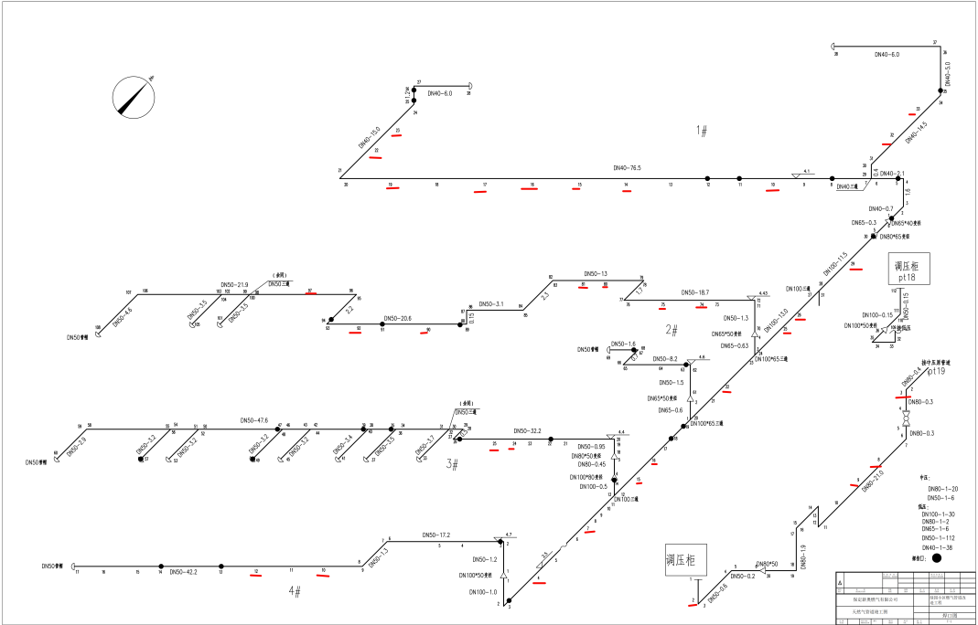
焊缝 焊缝-23
