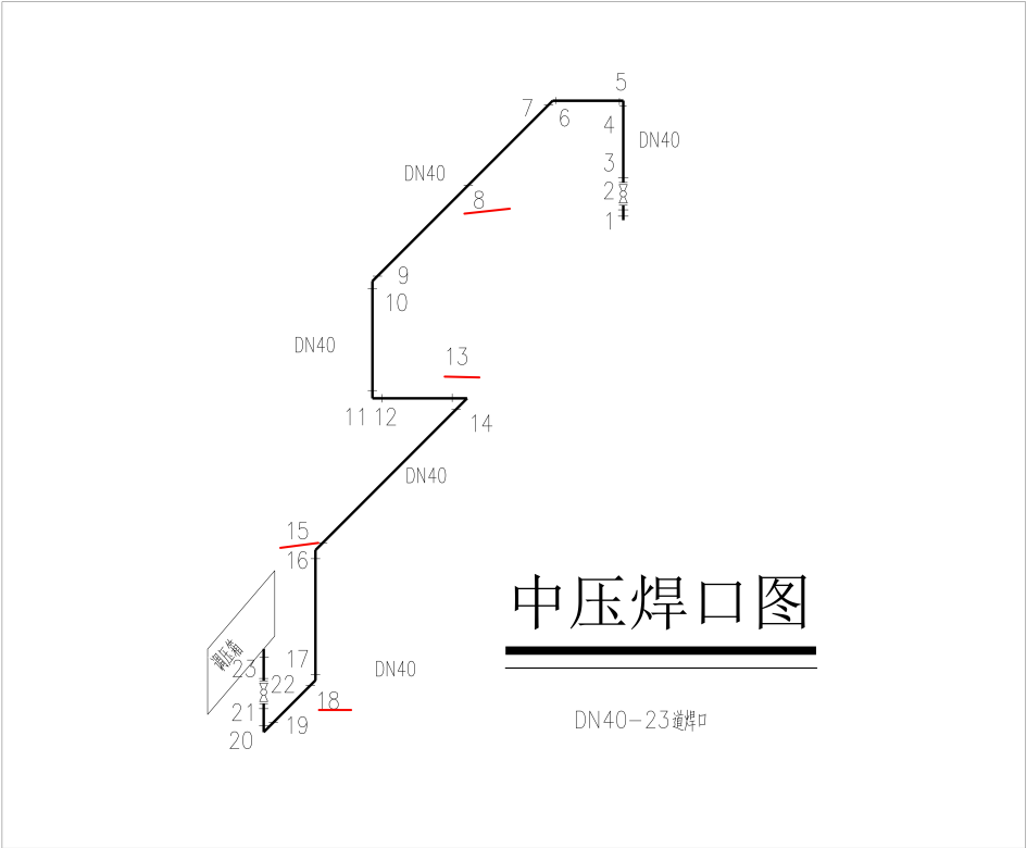
焊缝 焊缝-37
