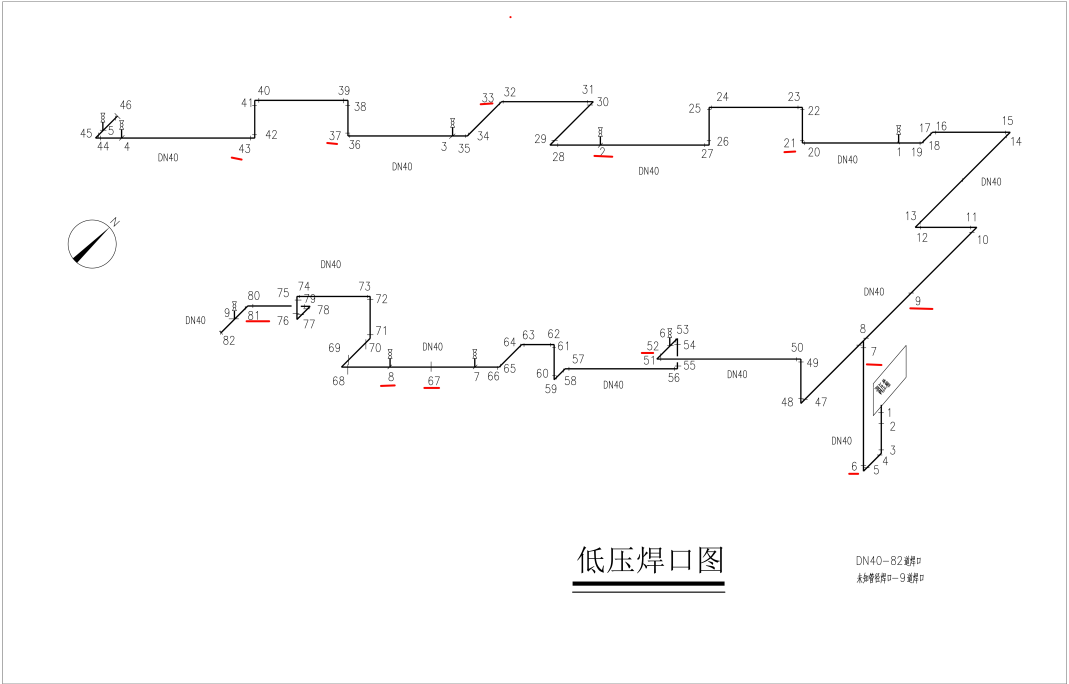
焊缝 焊缝-43
