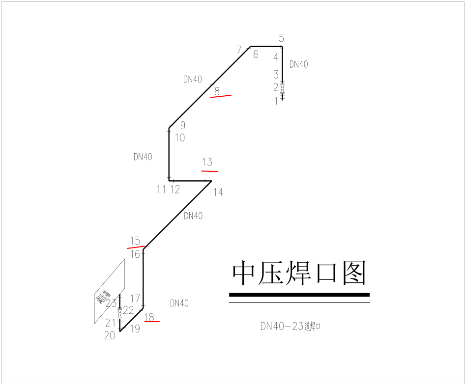
焊缝 焊缝-37
