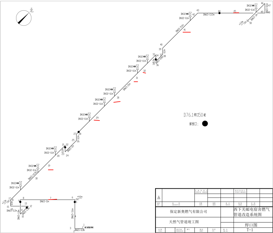
焊缝 焊缝-45
