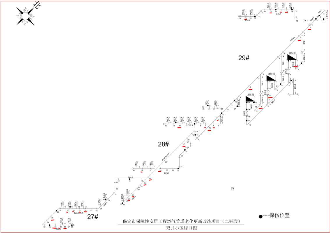
焊缝 焊缝-25
