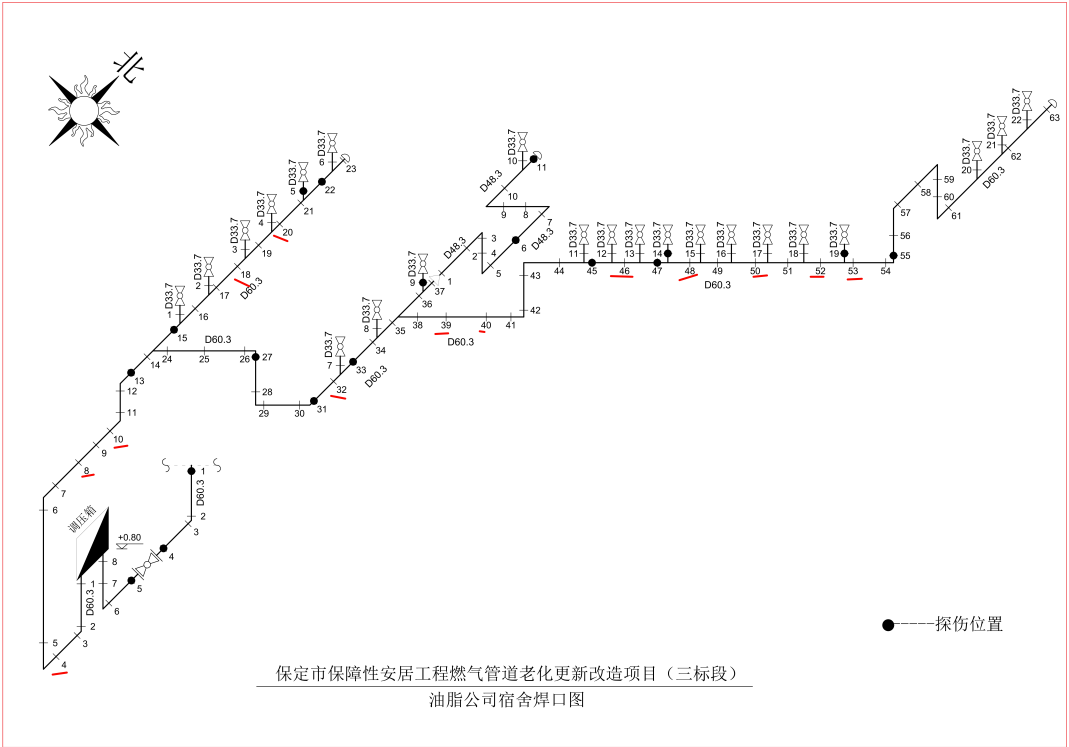
焊缝 焊缝-4
