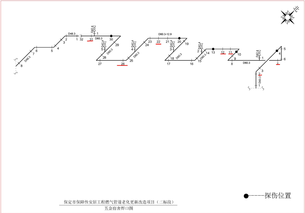
焊缝 2
