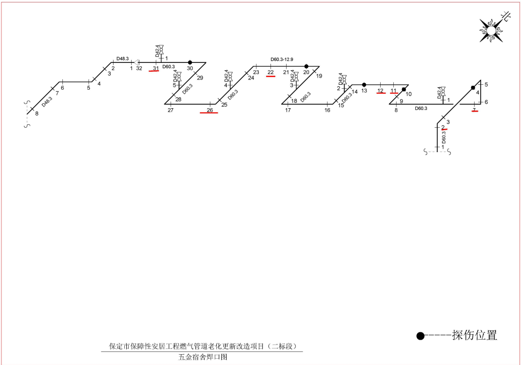
焊缝 7
