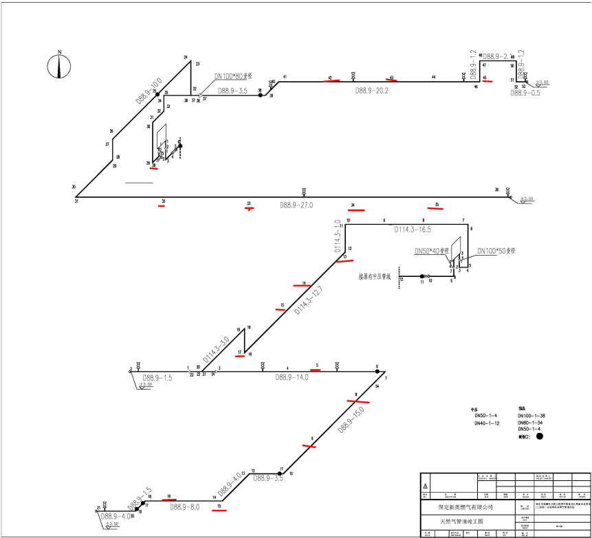
焊缝 45
