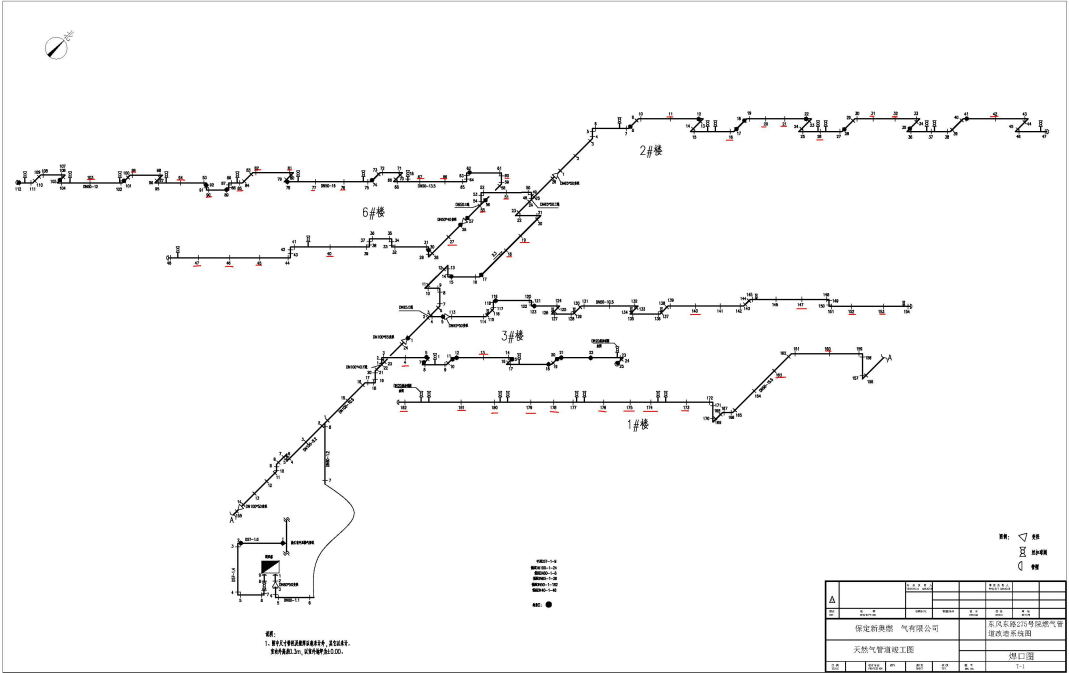
焊缝 103
