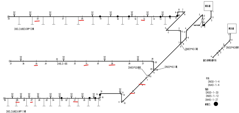
保百宿舍焊口图
