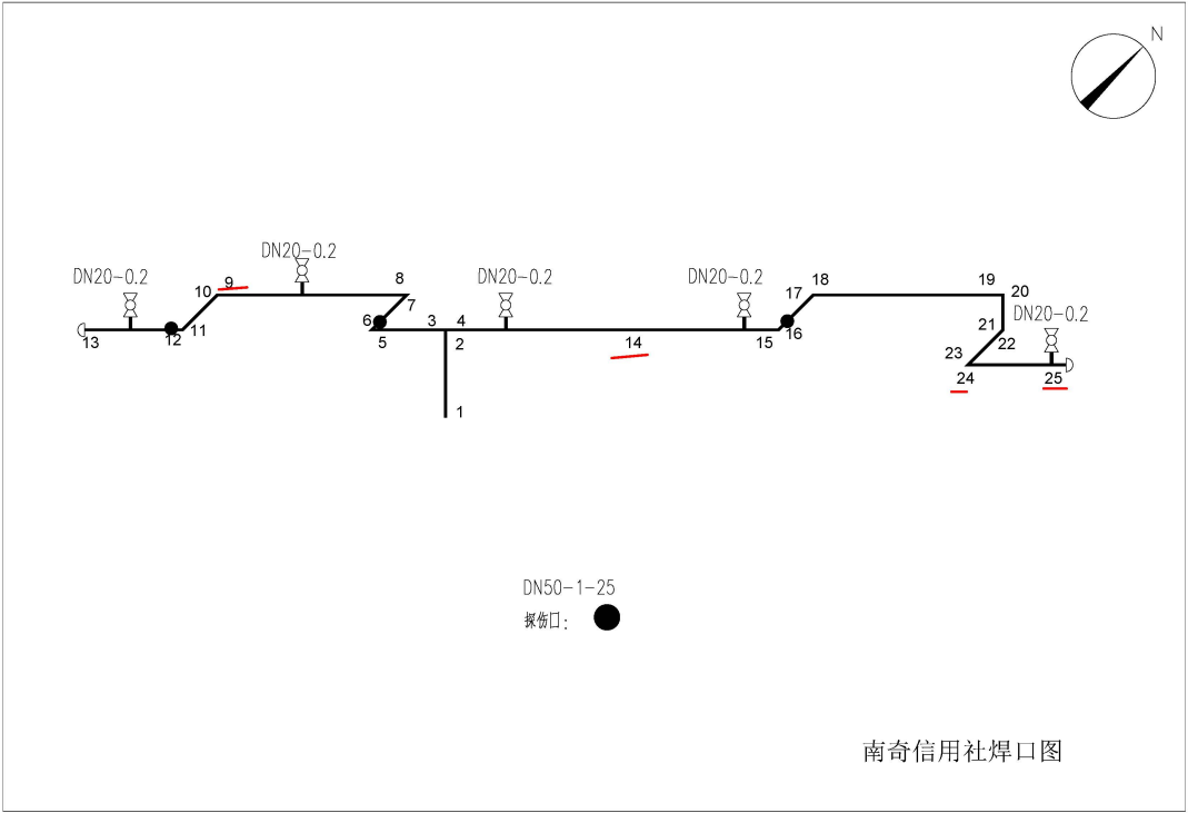
焊缝 9
